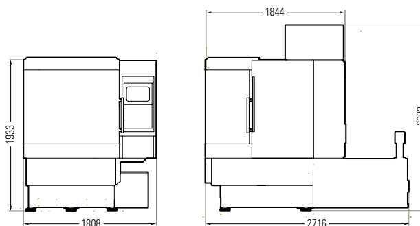
HELITRONIC ESSENTIAL (Rozměry jsou uvedeny v mm)
